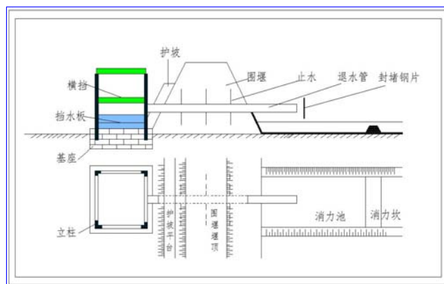
图1 退水口结构示意图
